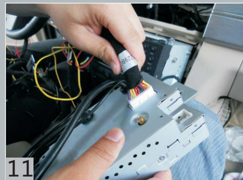
Подсоедините проводку к новому головному устройству.
