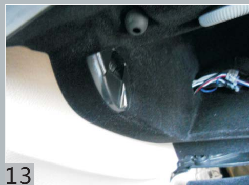
Протяните проводку для DVD плеера и провода USD в перчаточное отделение, соединив их вместе, как показано на фото.
